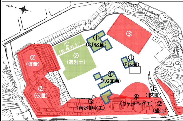
② 選別土仮置・盛土工 E工区、I区画の盛土を行っています。
