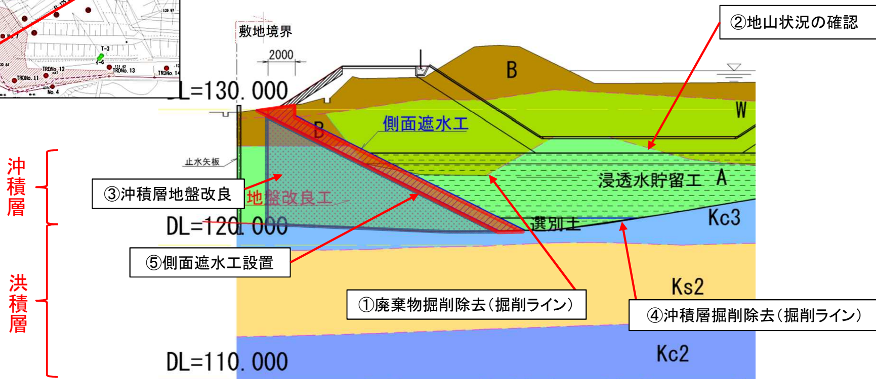
断面 R+15 (模式図)
