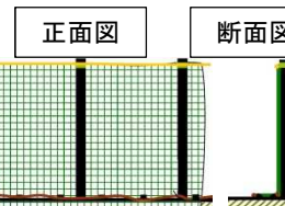
獣害防護柵構造図
