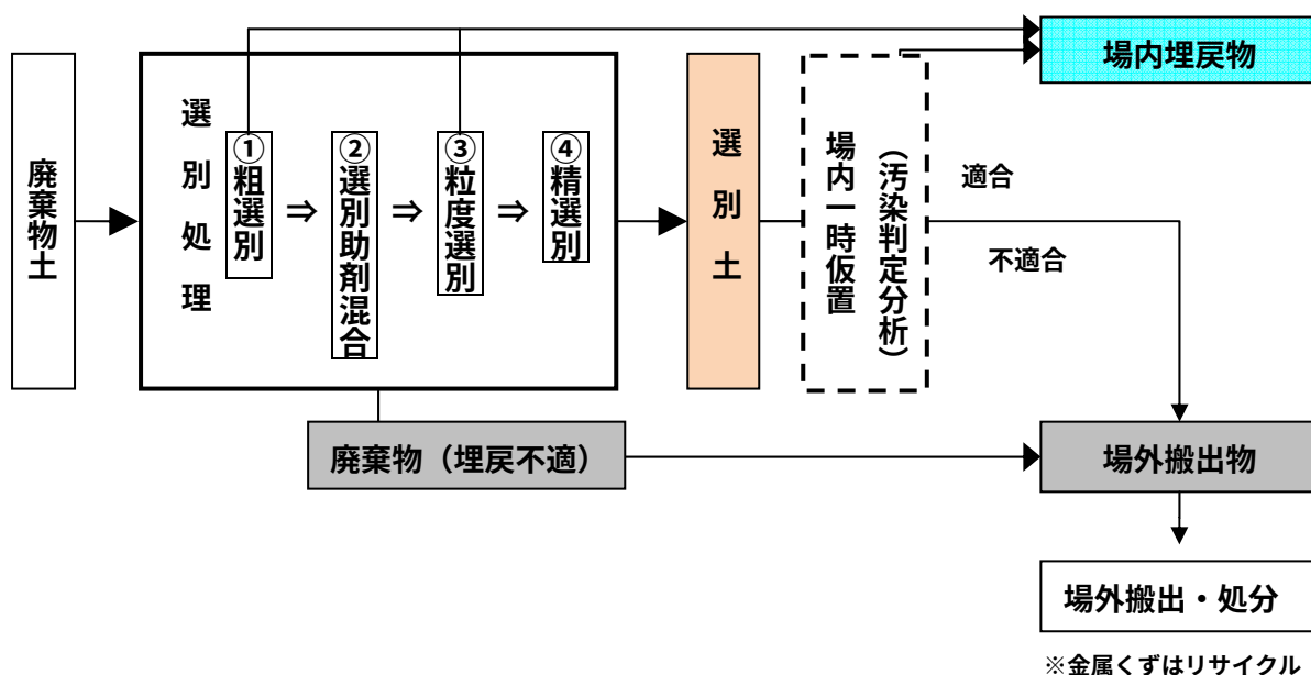
図3-5 廃棄物土の現場内処理と場外搬出のフロー
