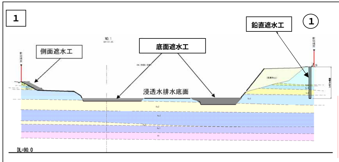
図 3-10 遮水構造図（ 1 - ①断面図）
