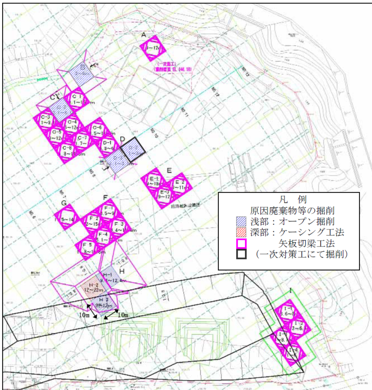
図 3-1 原因廃棄物等の掘削平面図
