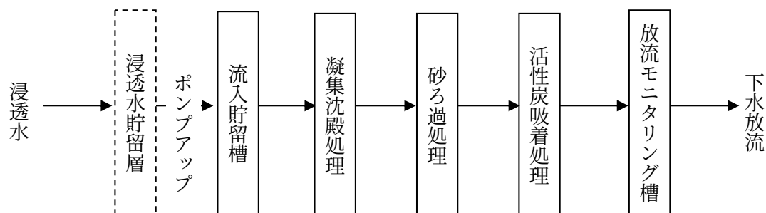
図 3-8 新設水処理施設処理フロー
