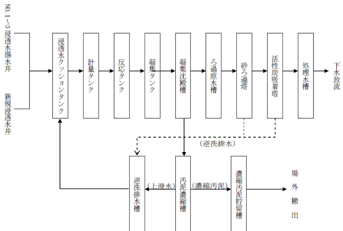
図 3-6 既設水処理施設ならびに No.1~3 浸透水揚水井 および新設浸透水揚水井
