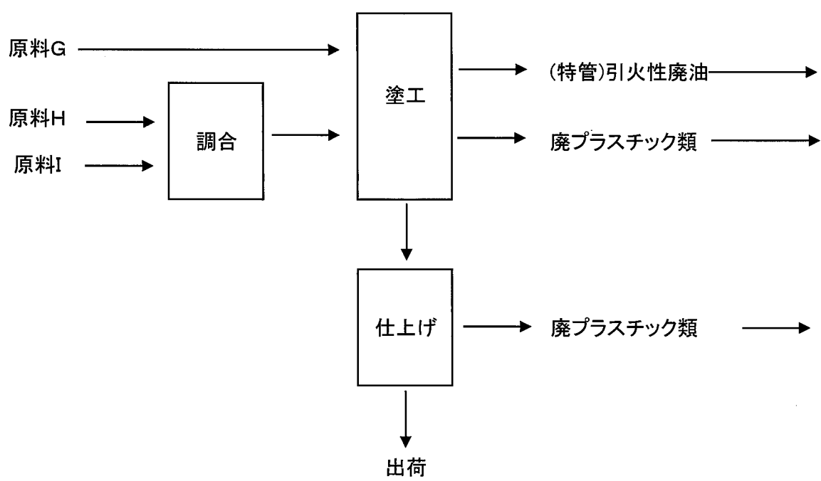
フィルム製造フロー図
