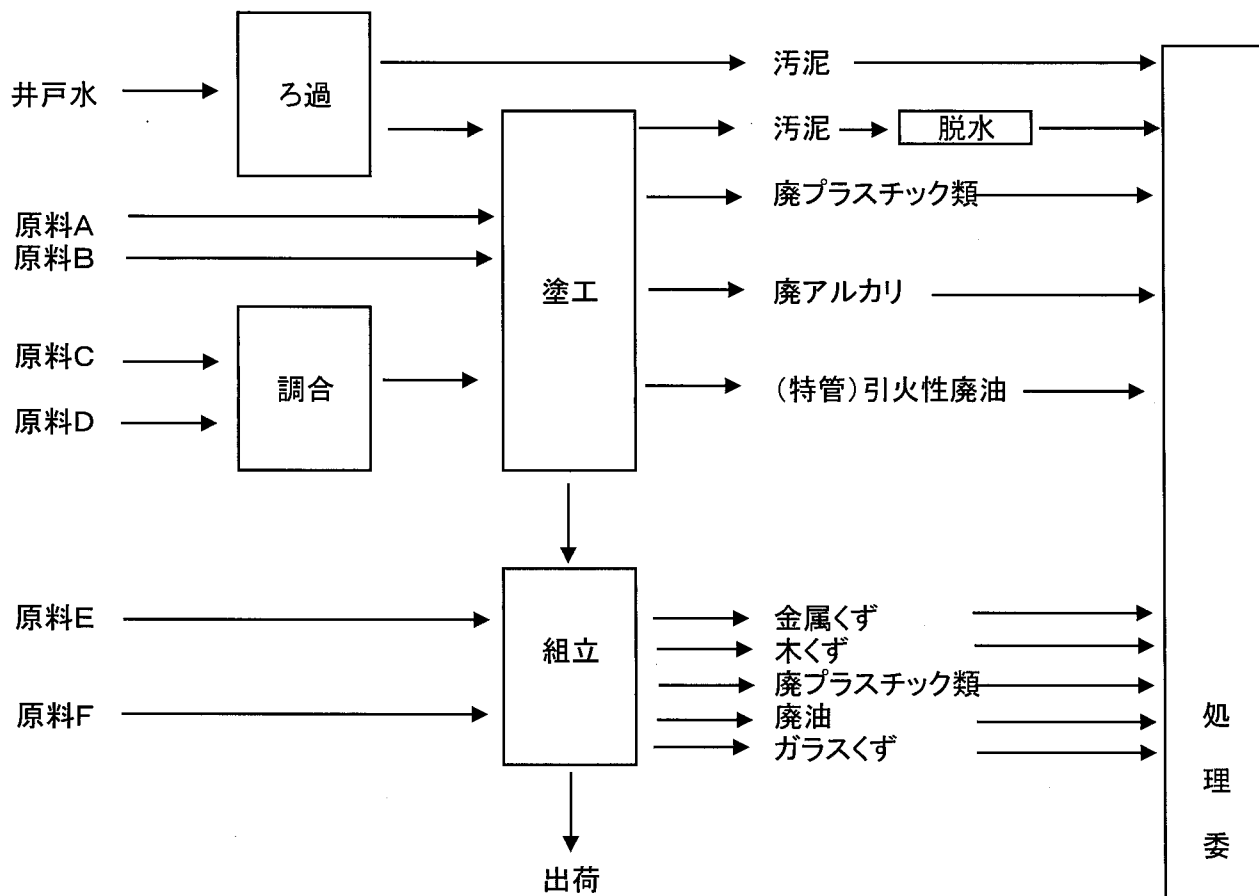
高分子ろ過膜製造フロー図
