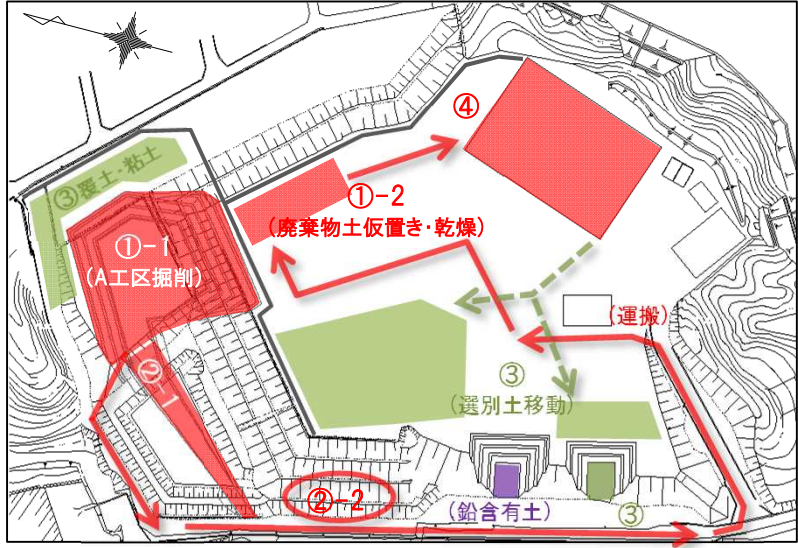
②-1 廃棄物土掘削工 A工区で従来のダンプ進入路を掘削しています。この後、新しい進入路に鉄板を敷きます。
