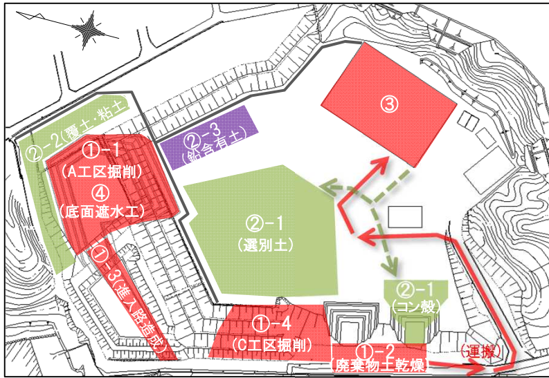
①-1 A工区掘削 止水矢板の内側を掘削しています。
