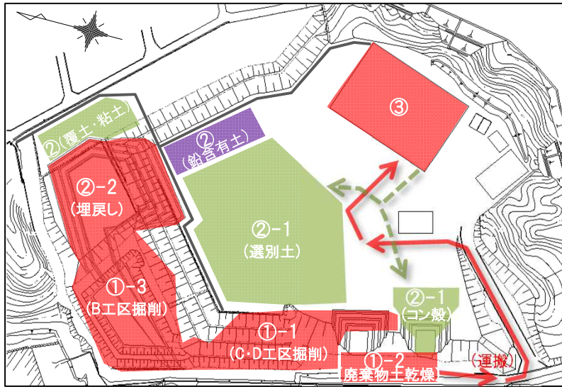
①-3 B工区掘削 B工区廃棄物土を掘削しています。
