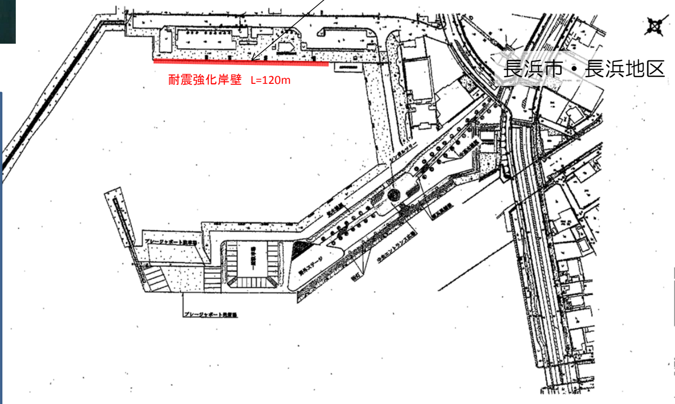
計画平面図
