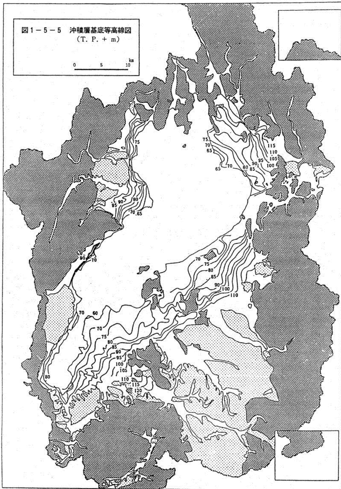
圖 1-5-5 沖積層基底等高線圖
