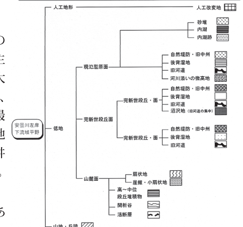
図5-1-1 安曇川左岸下流域平野の発達史的地形分類予察図とその凡例 (宮本, 2004を一部改変)
