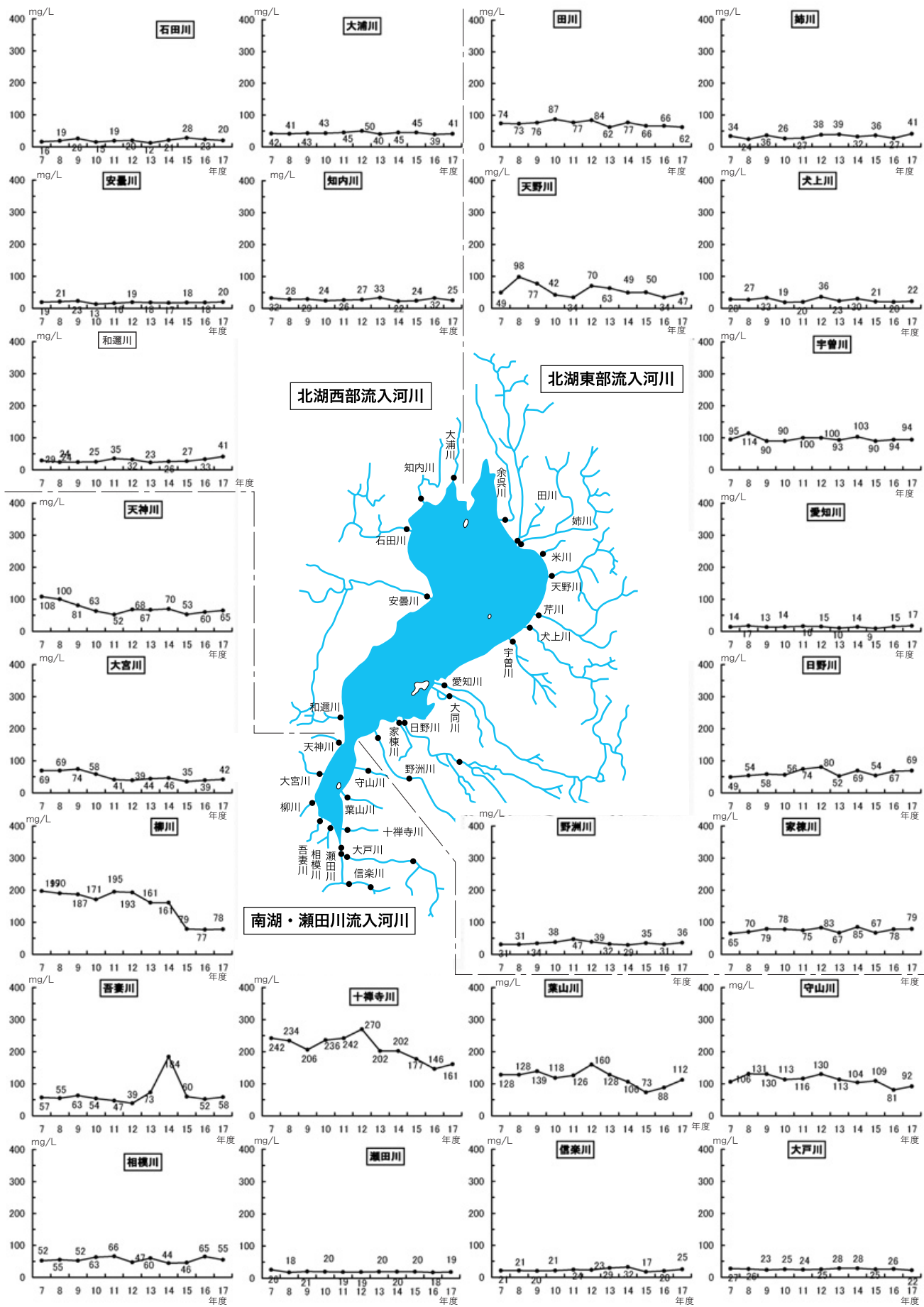
図(22)-4 環境基準点における全リン濃度の年間平均値の推移
