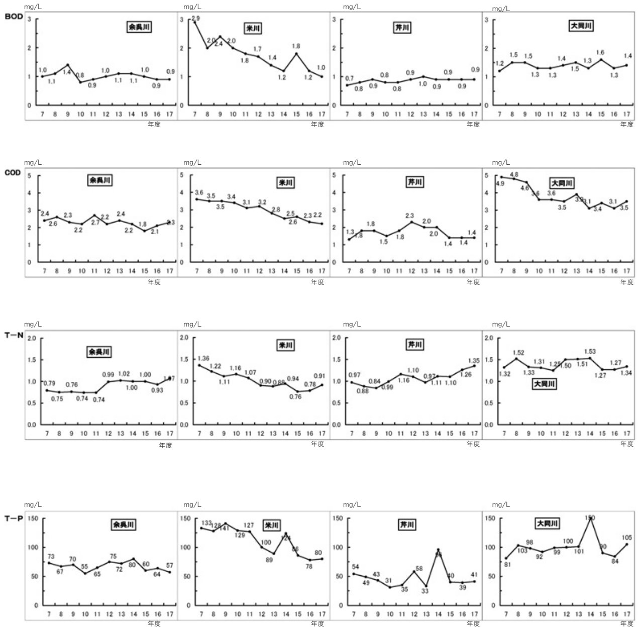
図(22)-5 環境基準未設定河川の水質状況
