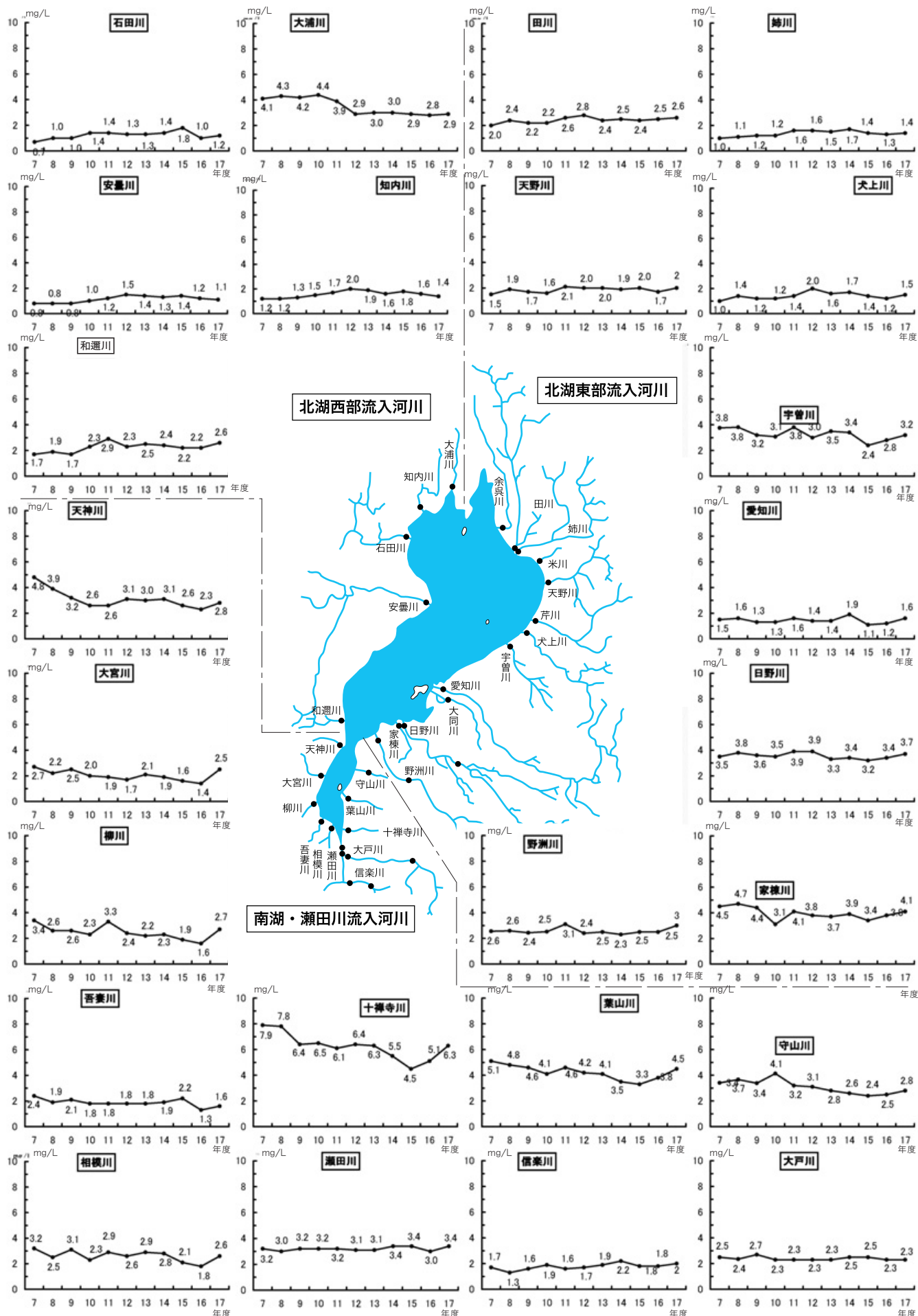
図(22)-2 環境基準点におけるCOD濃度の年間平均値の推移
