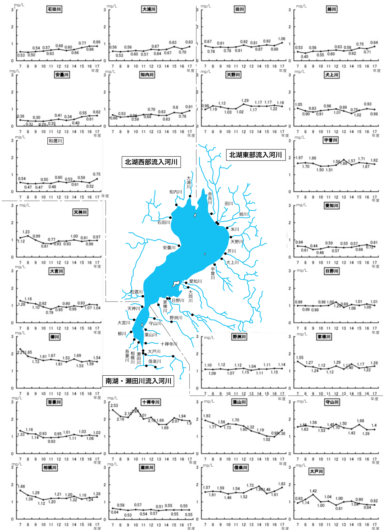
図(22)-3 環境基準点における全窒素濃度の年間平均値の推移
