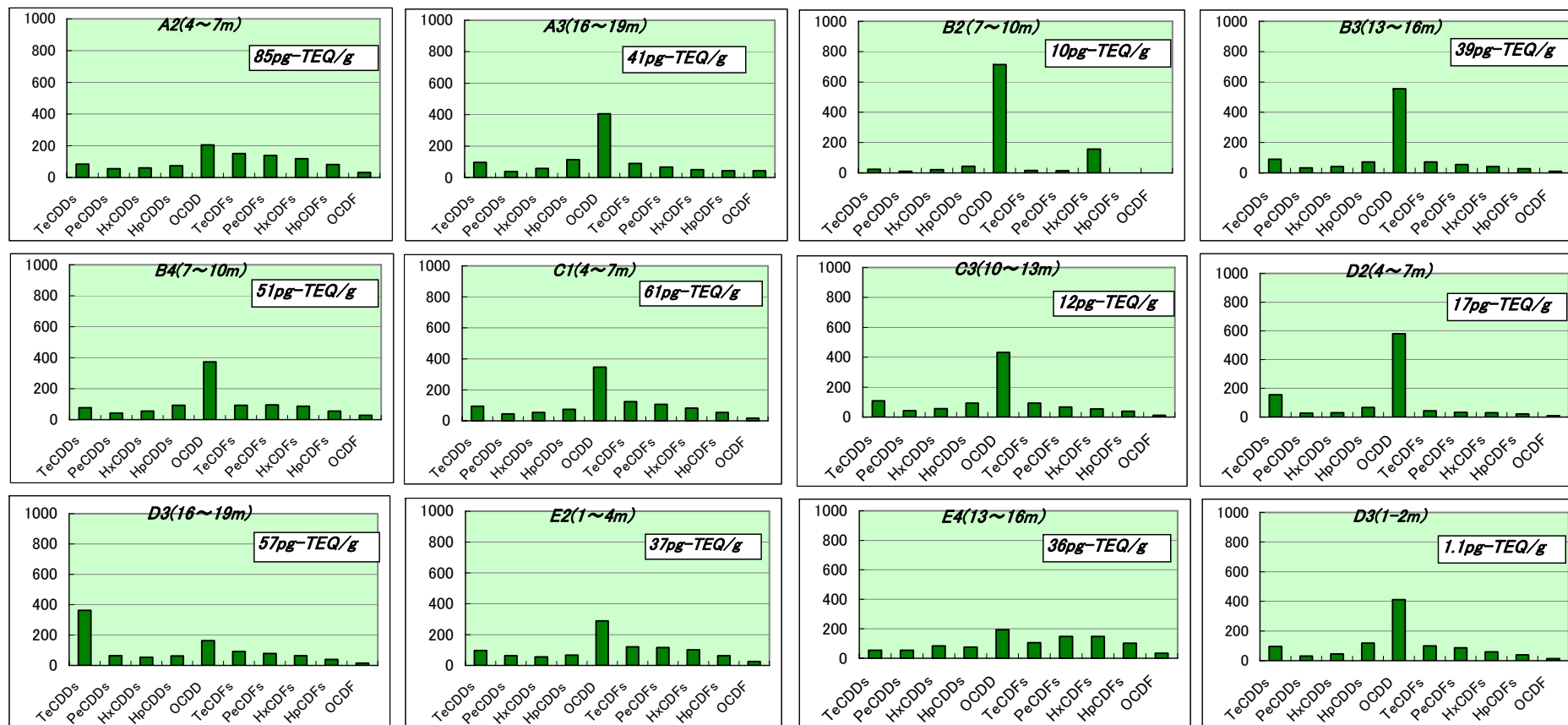
処分場内廃棄物土のダイオキシン類のパターン図(パターンは同族体実測濃度換算(%))。濃度は毒性換算濃度。)
