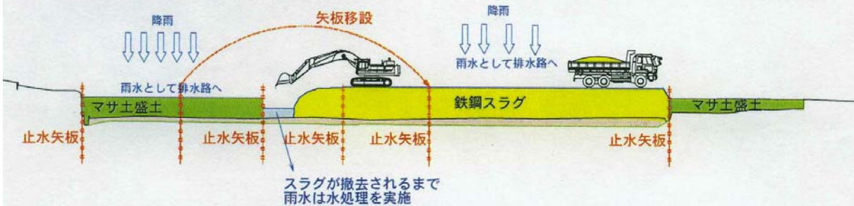
③矢板を設置しての第3工程(エリア3撤去) 矢板移設
