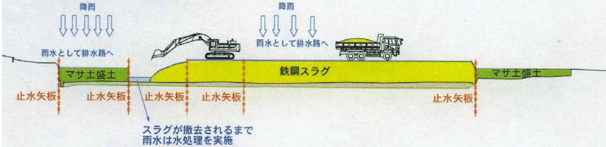
②矢板を設置しての第2工程(エリア2撤去)
