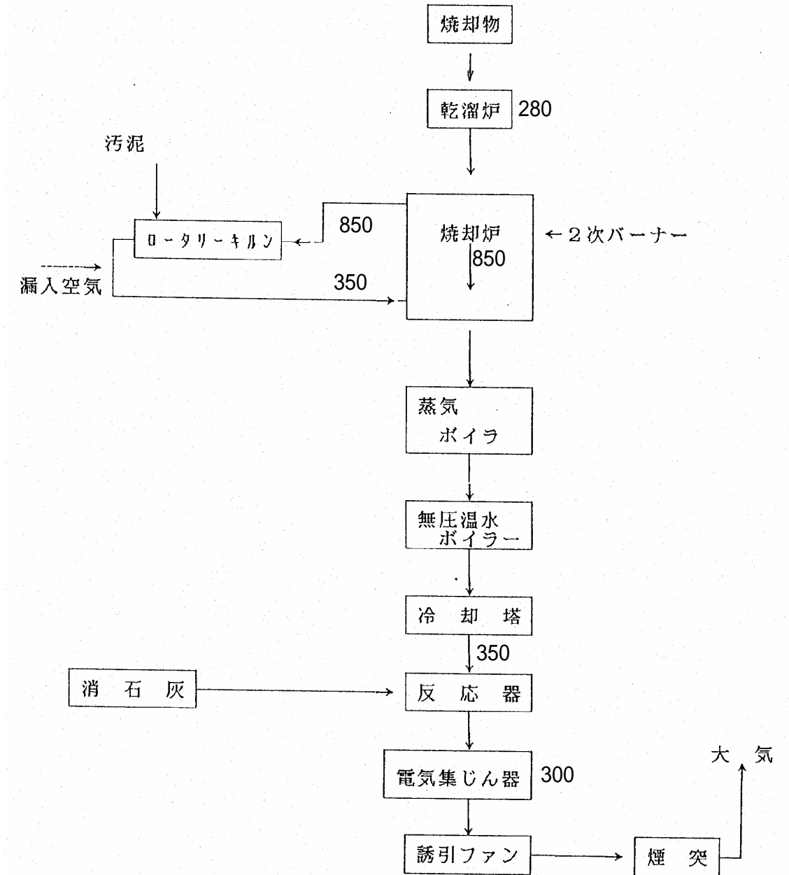
図2.2 南側焼却炉フローシート（設計計算時の設定温度）
