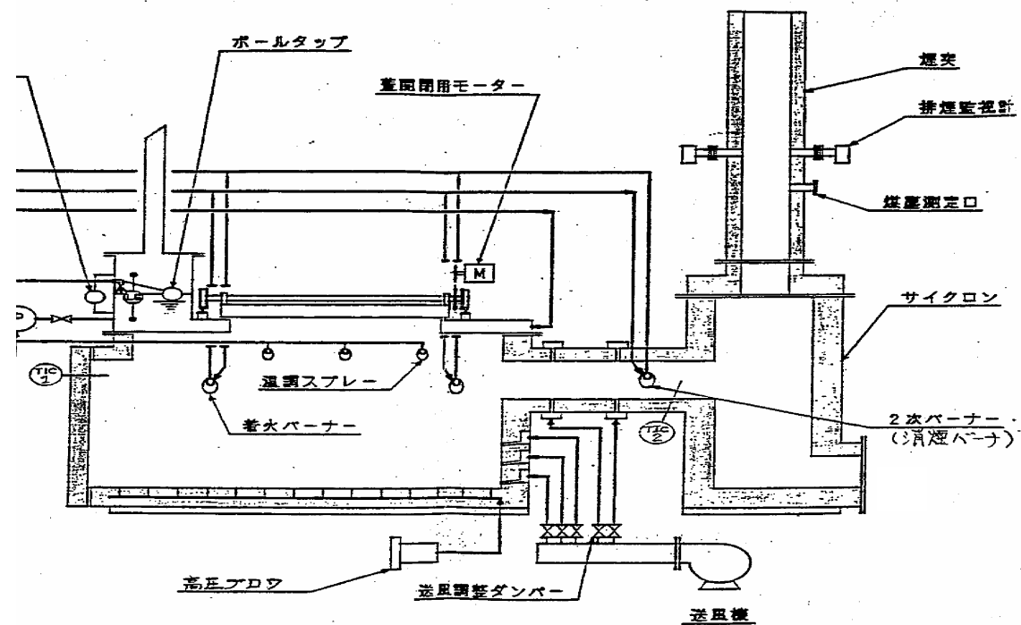
図 2.3 東側焼却炉フロー図
