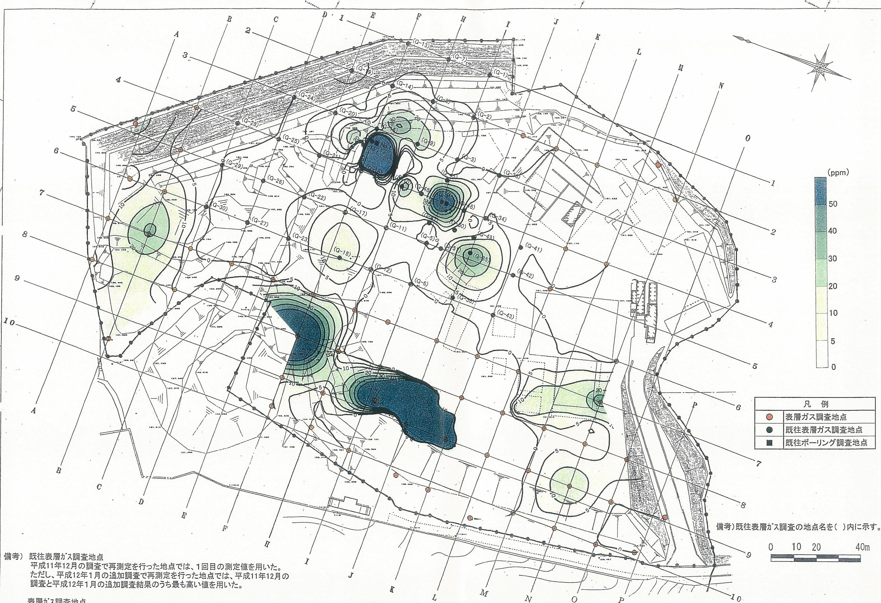
図3-1(4) 表層ガス濃度等高線図(硫化水素)
