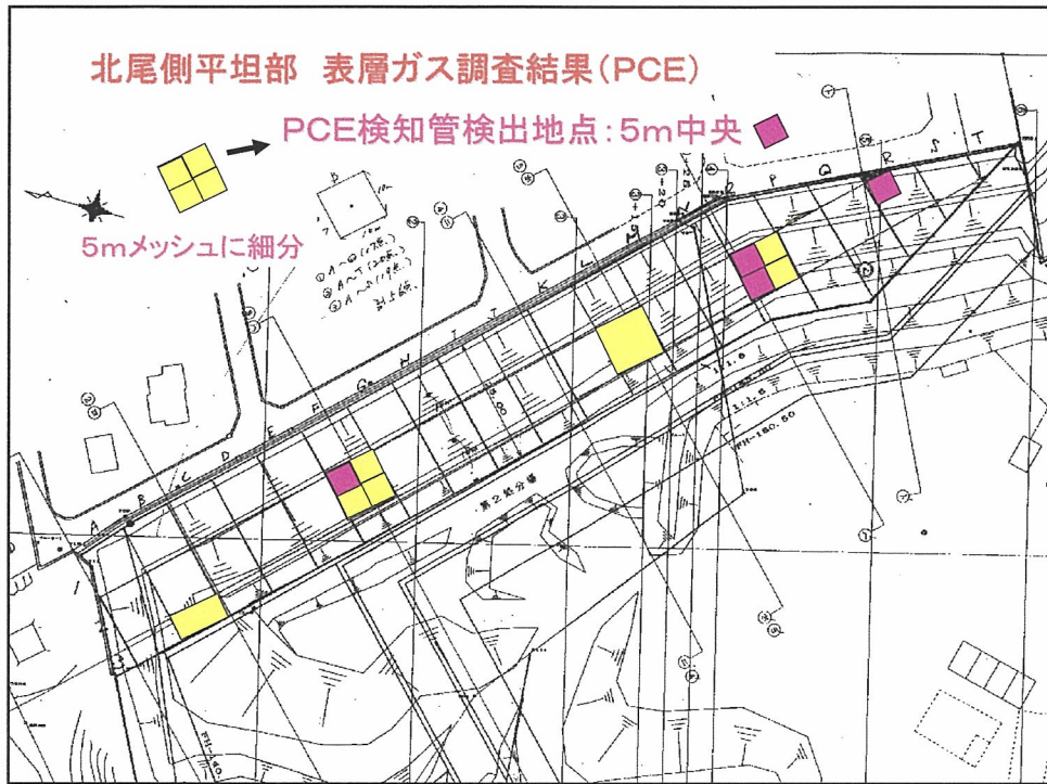
図2.6-10 北尾側平坦部 表層ガス調査結果(PCE)
