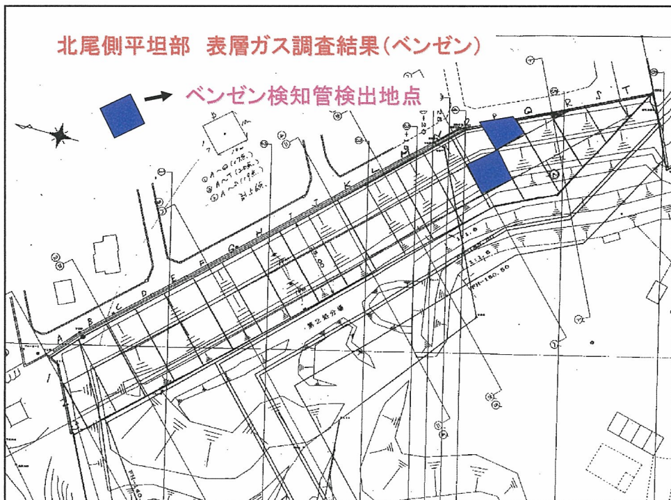
図2.6-11 北尾側平坦部 表層ガス調査結果(ベンゼン)
