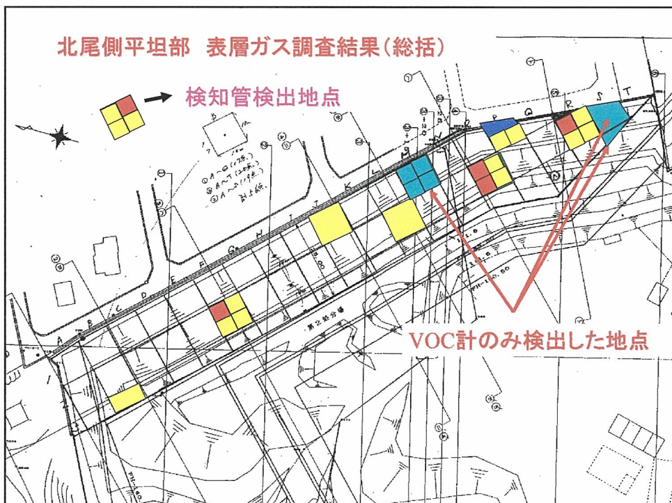
図2.6-13 北尾側平坦部 表層ガス調査結果(総括)
