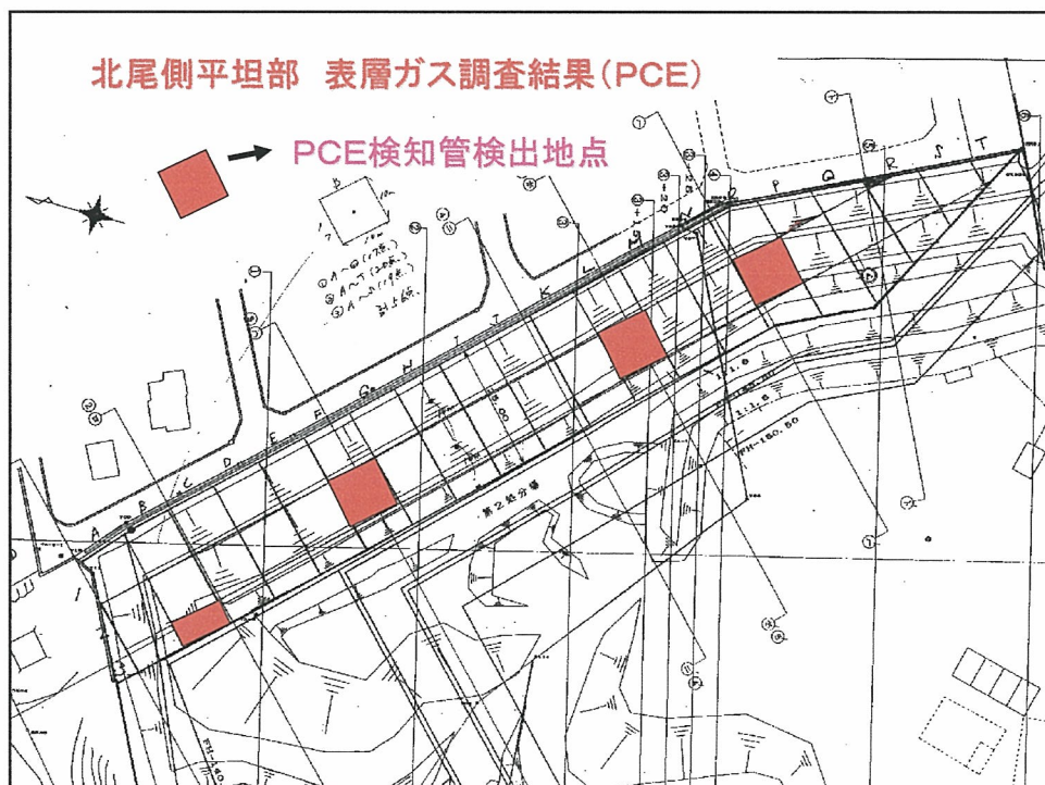
図2.6-9 北尾側平坦部 表層ガス調査結果(PCE)
