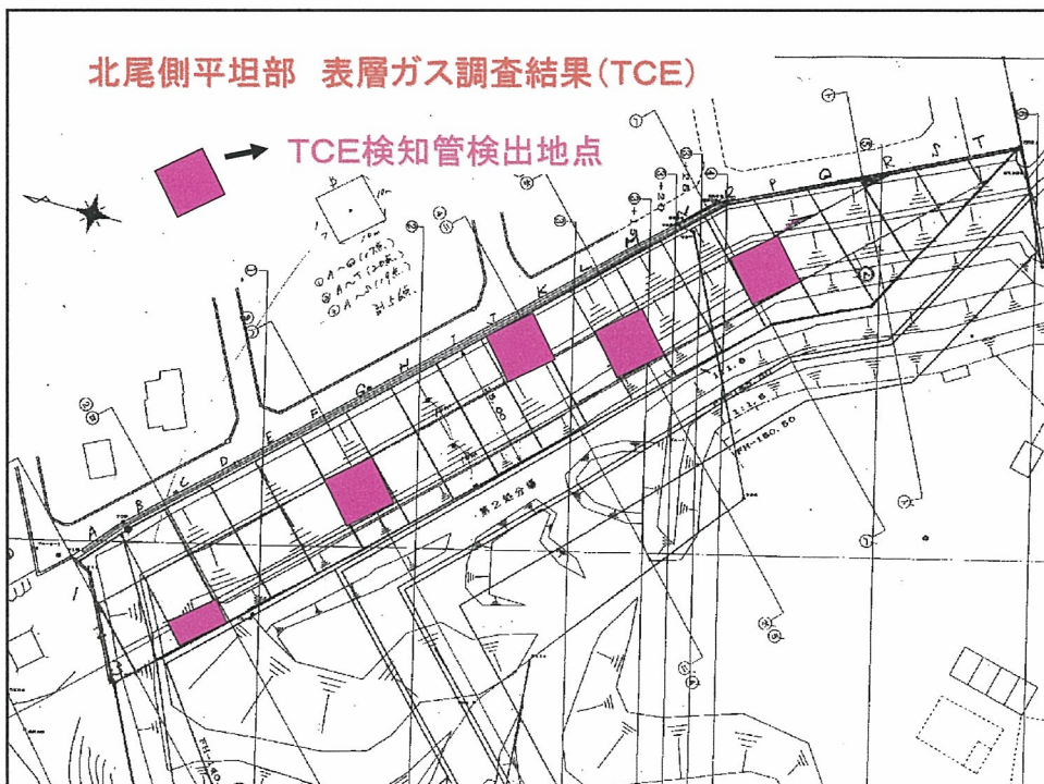
図2.6-7 北尾側平坦部 表層ガス調査結果(TCE)
