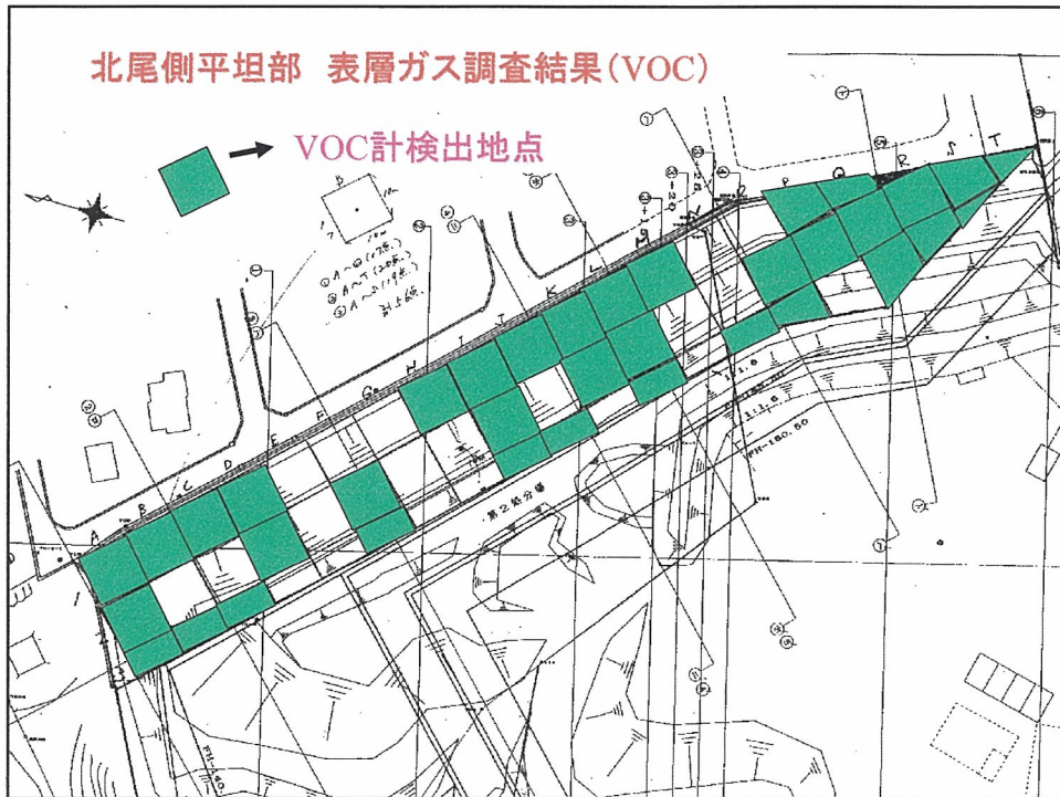
図2.6-6 北尾側平坦部 表層ガス調査結果(VOC)
