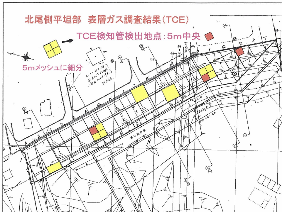
図2.6-8 北尾側平坦部 表層ガス調査結果(TCE)
