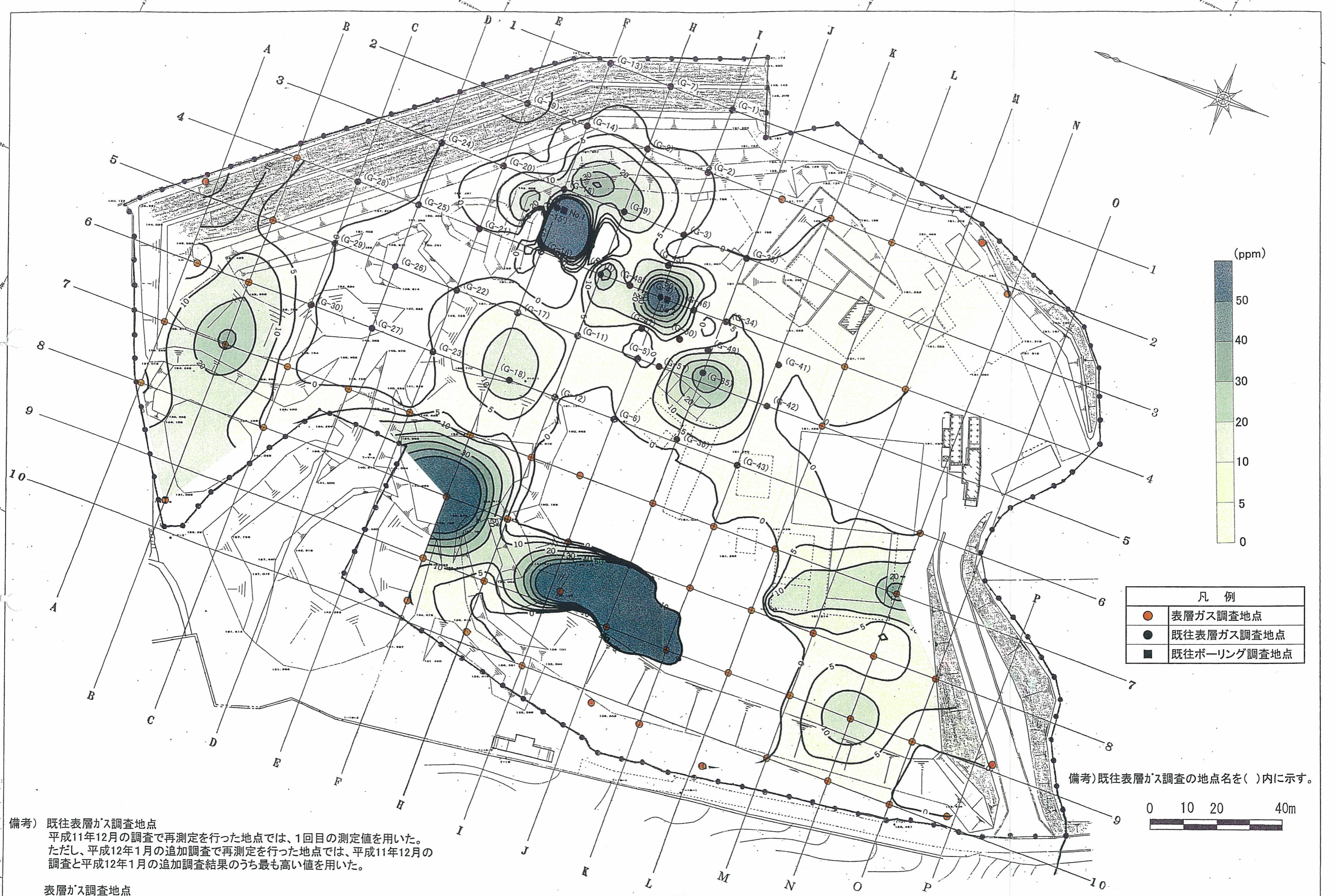
図2.6-4 表層ガス濃度等高線図(硫化水素)
