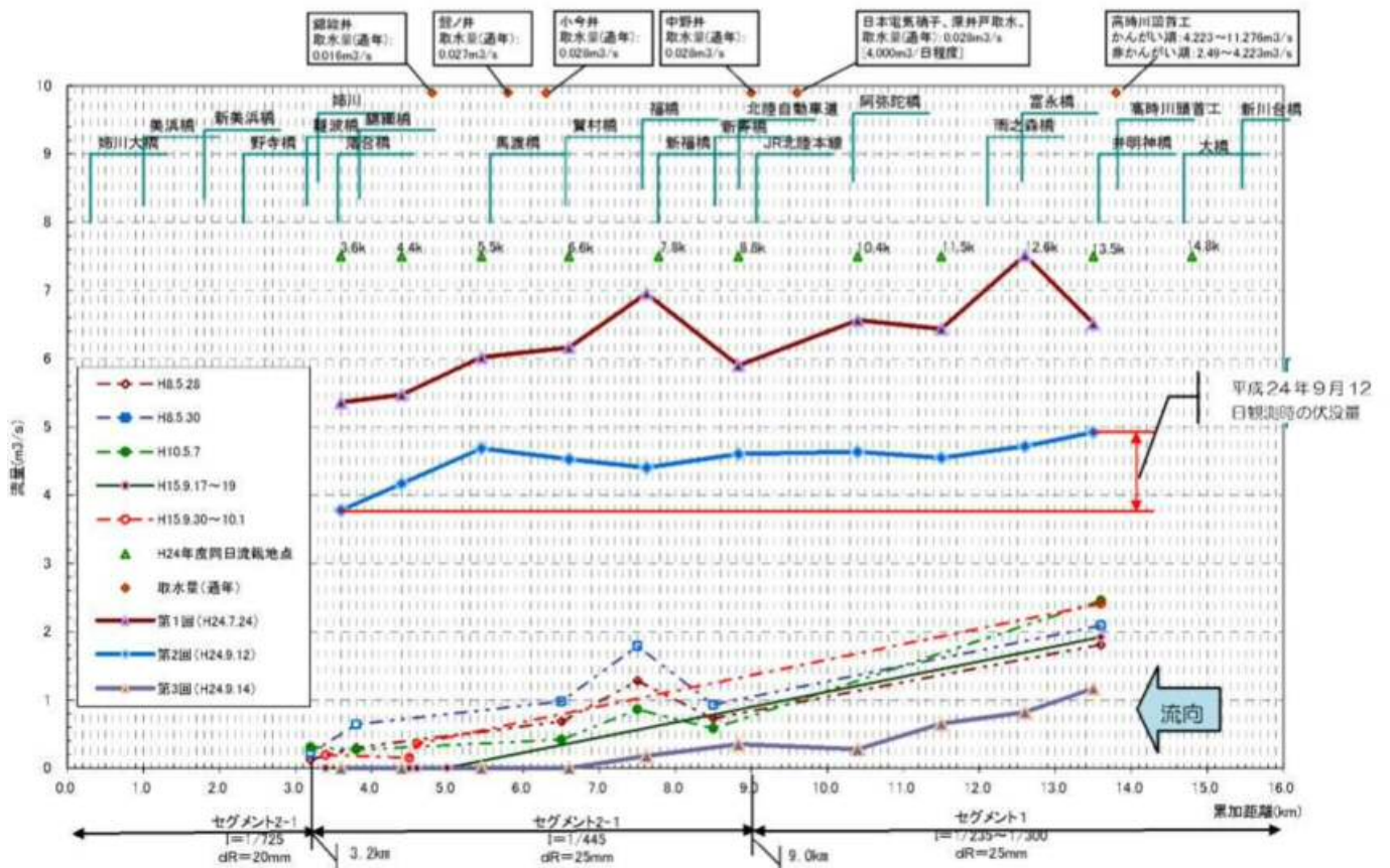
図 3.1 伏没量の縦断変化の整理例
