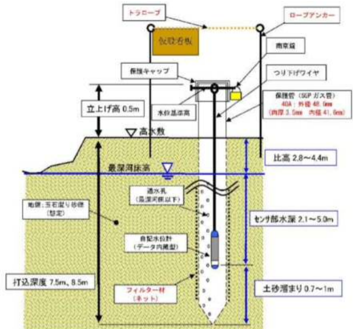
図 3.3 地下水位計設置例
