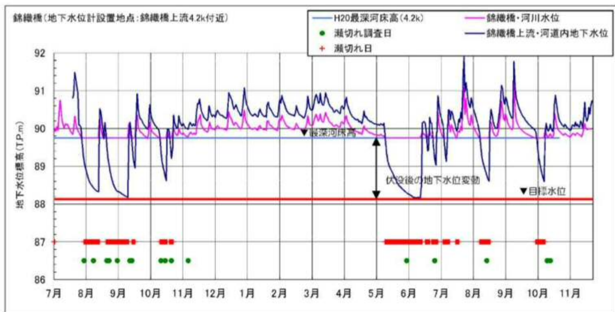
図 3.4 河道内地下水位観測例（高時川・下流錦織橋上流）
