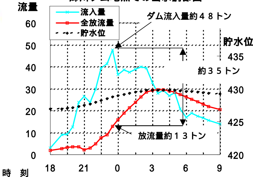
姉川ダム地点での出水調節図
