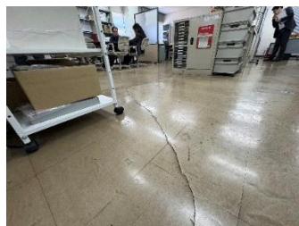
地盤沈下により建物周辺や建物内部に段差が発生
