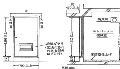
機械室の例
