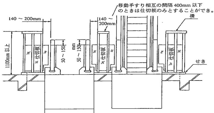
仕切板とエスカレーター各部とのすき間は100mm以下とする(上図参照)
