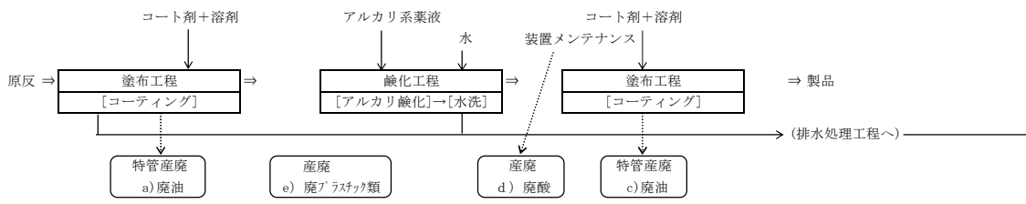
図4 調光フィルムの製造フローシート【No.4】
