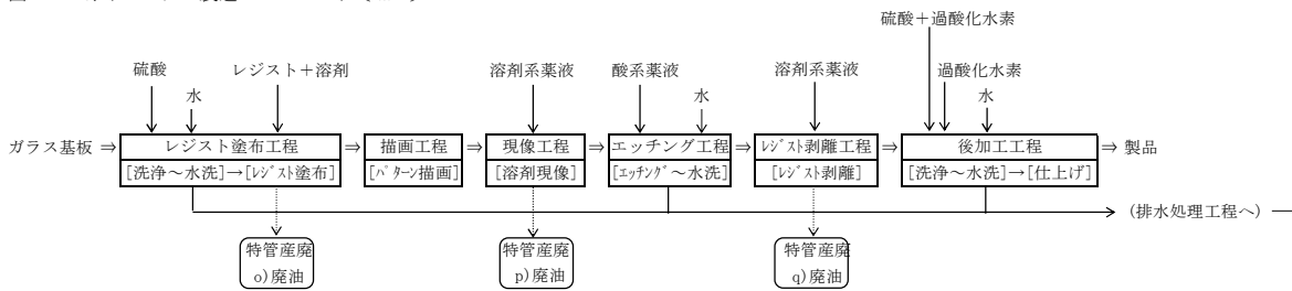
図3 反射防止フィルムの製造フローシート【No.3】
