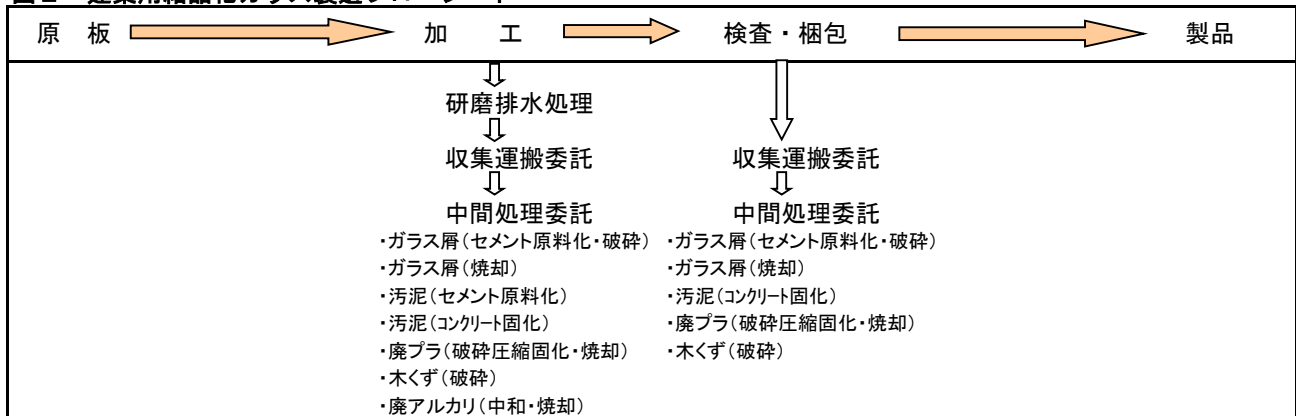
図2 建築用結晶化ガラス製造フローシート
