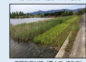
底質改善対策（覆土工・植生工）
