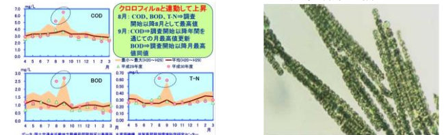
平成30年度南湖主要水質項目の経月変動（表層平均値） 平成30年夏季に南湖で大増殖した7ヶヶトナリ
