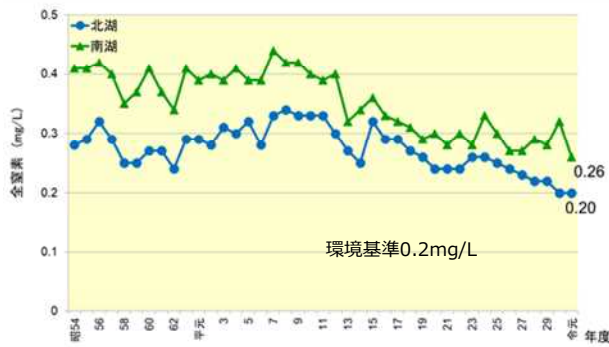
【図表3】全窒素
