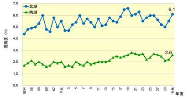
【図表2】透明度
