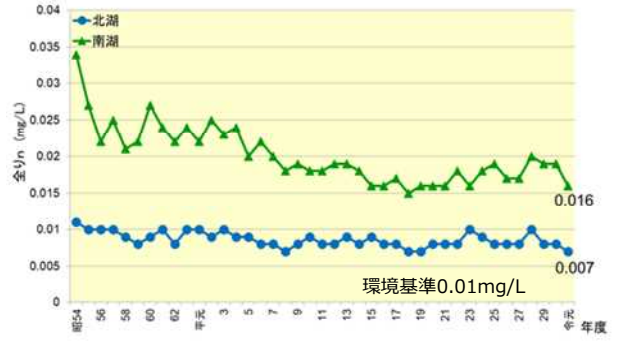
【図表4】全りん
