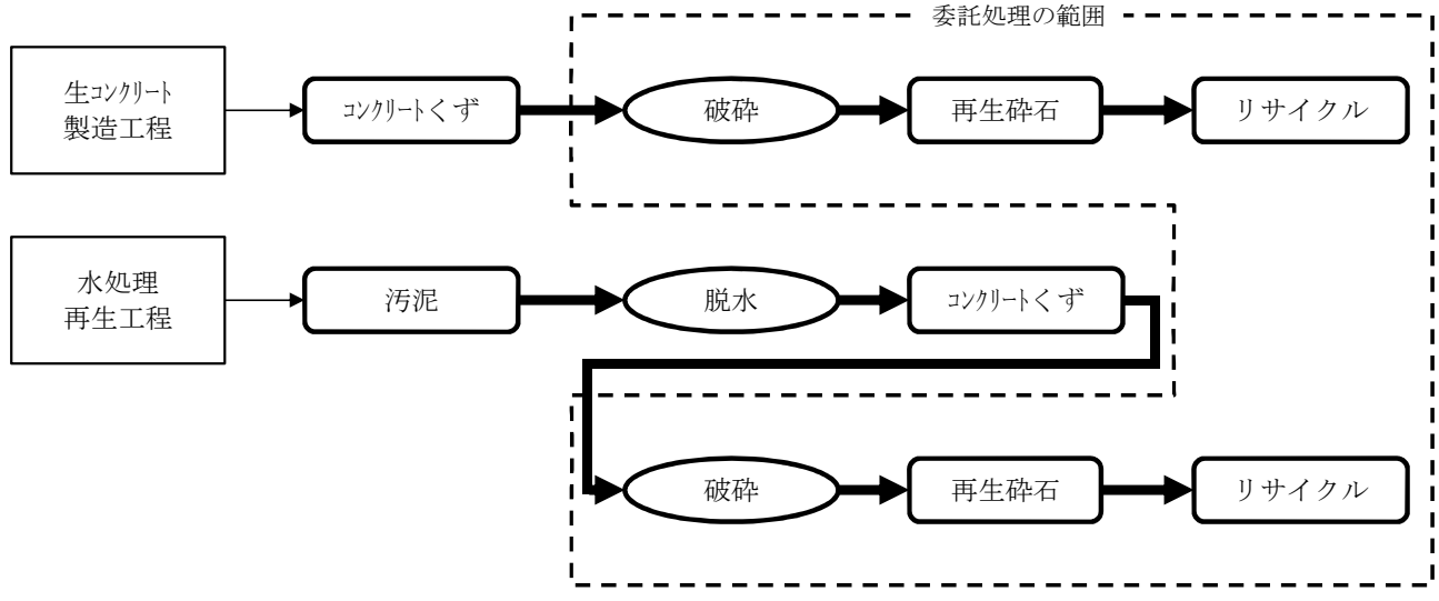
別紙 産業廃棄物の一連の処理の工程
