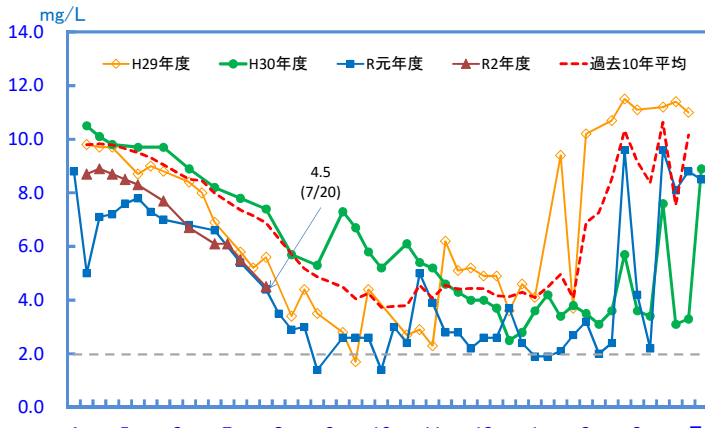
【図表12-6】北湖代表点（今津沖中央）における底層DOの経月変動
