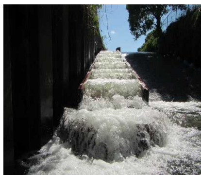
【図表7-3】2019年度に設置した際の魚道 【図表7-4】ピワマスが魚道を遡上している姿（「家棟川・童子川・中ノ池川にピワマスに戻すプロジェクト」提供）
