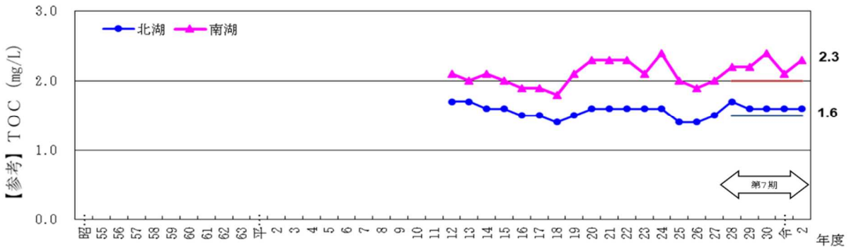
図2 水質の経年変化（— は各計画期間の目標値を示す）
