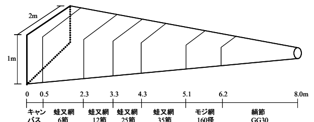
図4 角形幼生網
