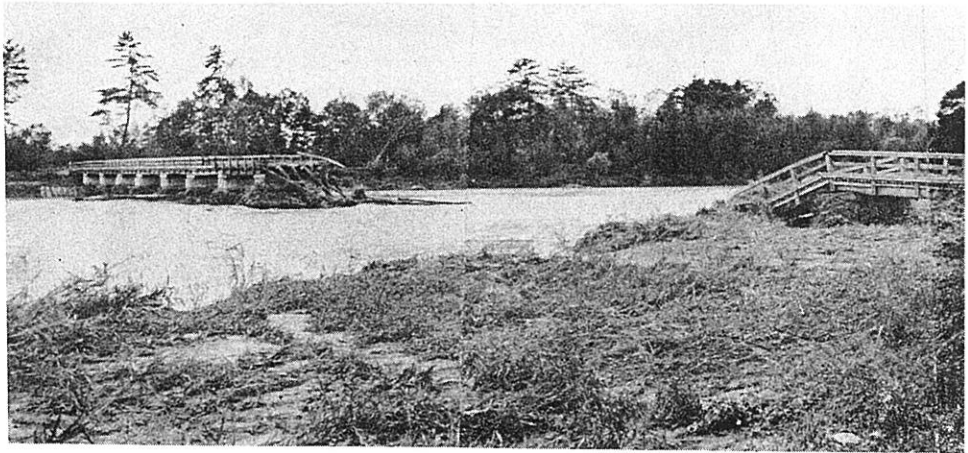
宮上橋の流失 (日野川)
