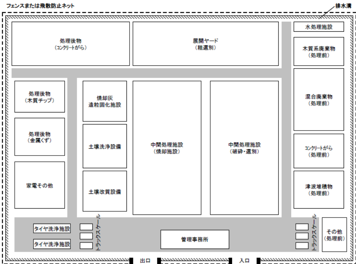
図表 62 二次仮置場レイアウト (例)
