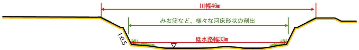
大戸川上流区間横断面図
