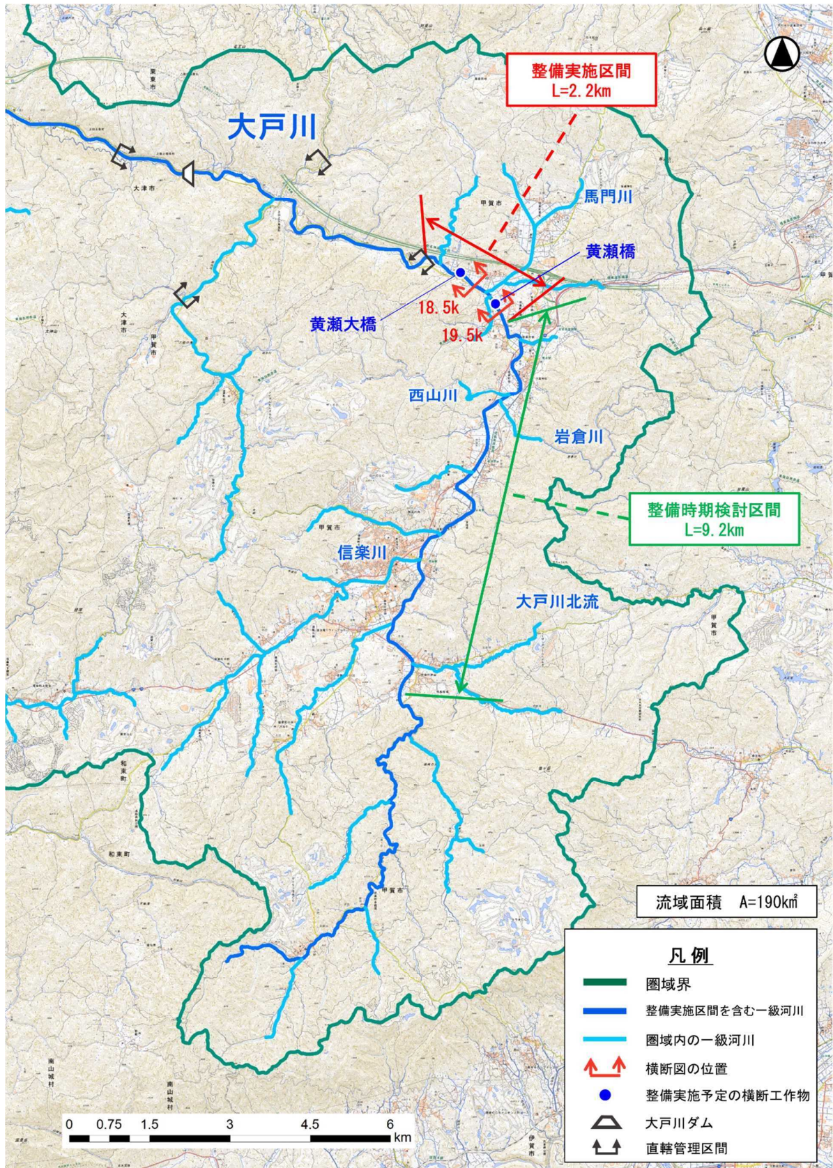
大戸川上流区間平面図
