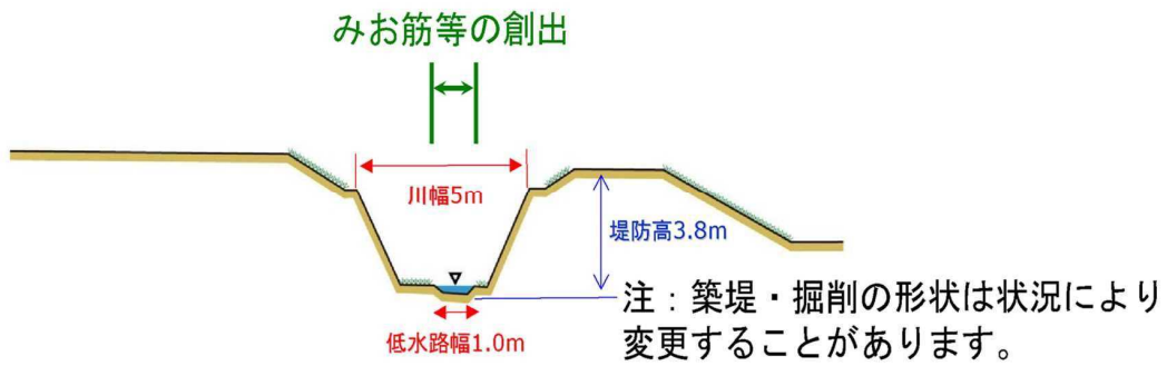
高橋川横断面図
