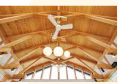
宮村さんが設計された、びわ湖材100%の屋根架構。木材を折れ線状につなげたアーチが特徴。(琵琶湖汽船 今津営業所)
