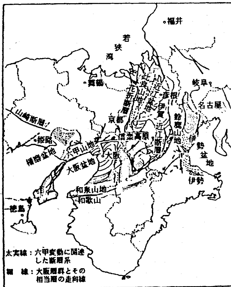
図 1-5-2 近畿三角地帯の地質構造図
