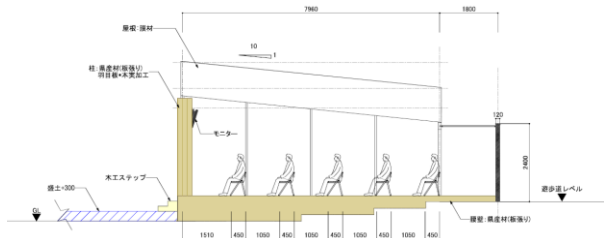
【側面図】
