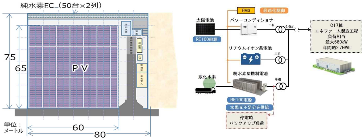
RE100 化ソリューション実証施設レイアウト
