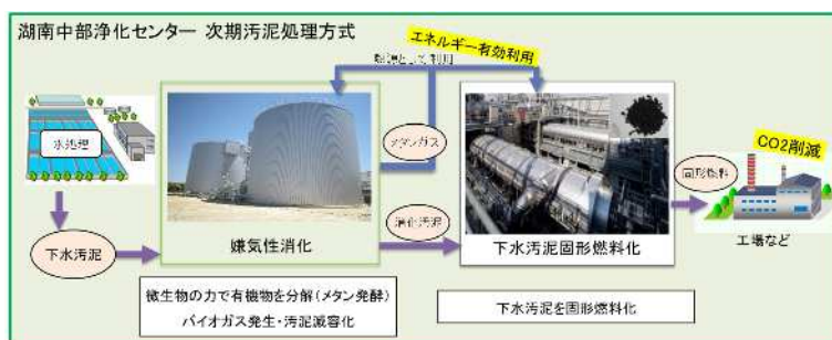
図 5-17 湖南中部浄化センターの次期汚泥処理方式概略図
