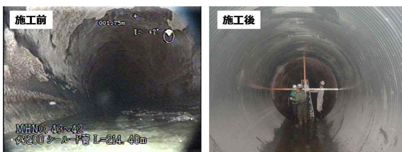
図 5-23 老朽化した下水道管の更生
