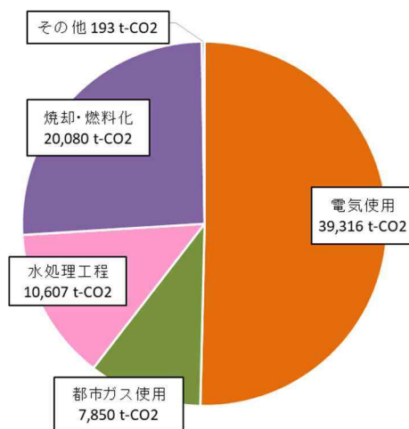
図 5-16 流域下水道温室効果ガス排出量内訳 (平成 30 (2018) 年度)
