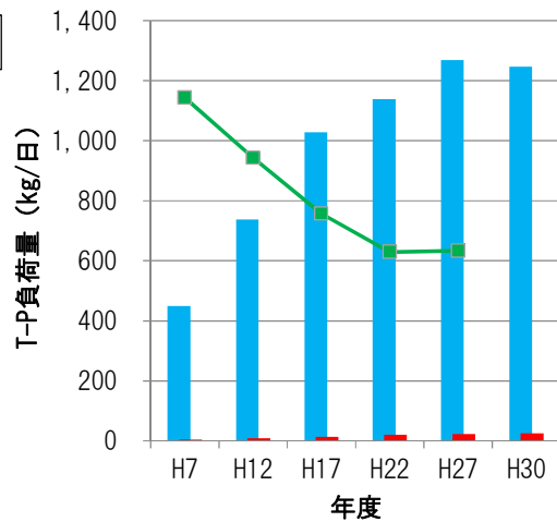
図 1-5 流域下水における負荷削減の経年変化
