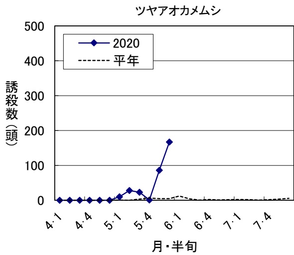
図1 フェロモントラップにおけるチャバネアオカメムシとツヤアオカメムシの誘殺数の推移（栗東市荒張）
