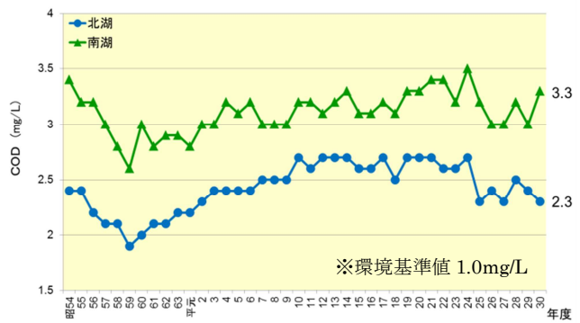
有機物 (COD)
