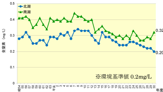
全窒素 (T-N)
