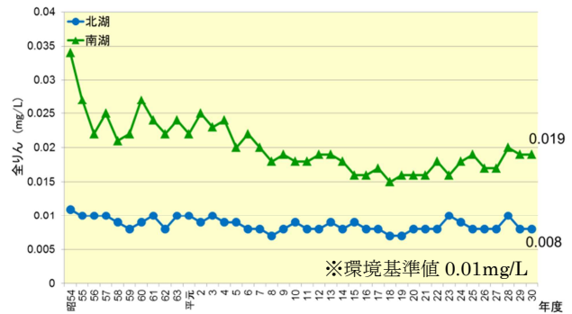
全りん (T-P)
