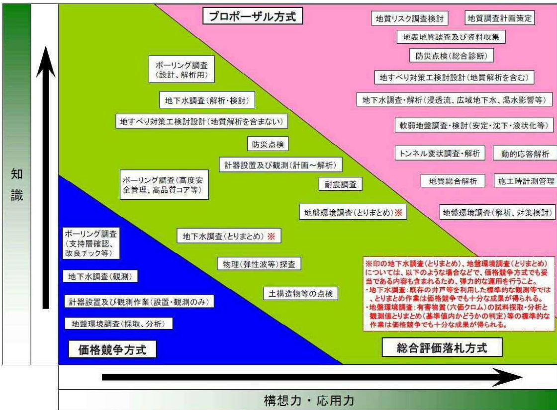
図-4 地質・土質調査の例
