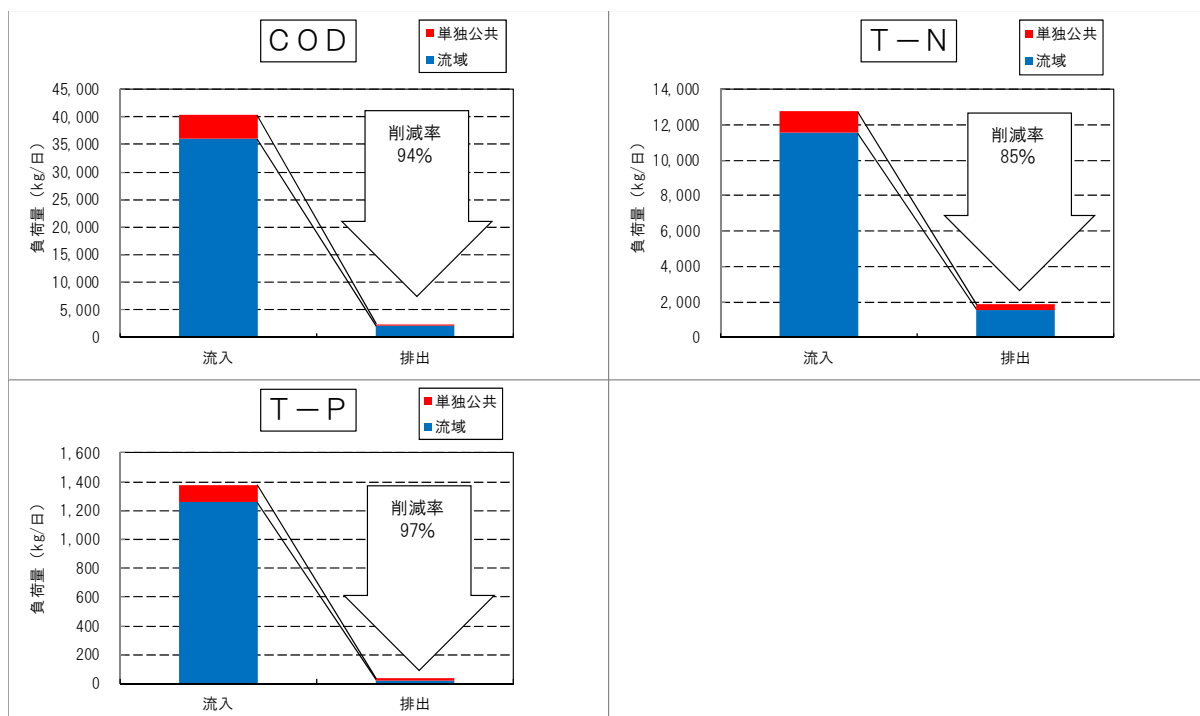
図 3-3-6. 滋賀県内の流域下水道処理場における汚濁負荷量削減状況 (H26)
