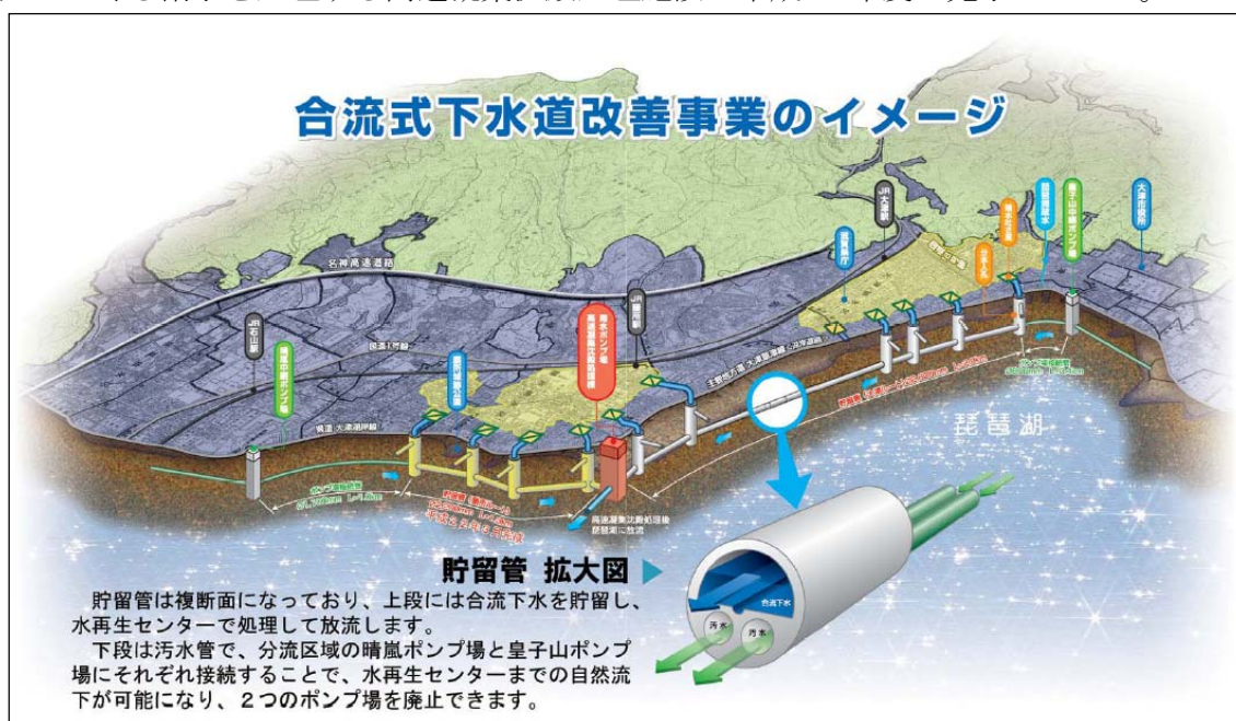
図 3-3-10. 合流式下水道改善事業イメージ
