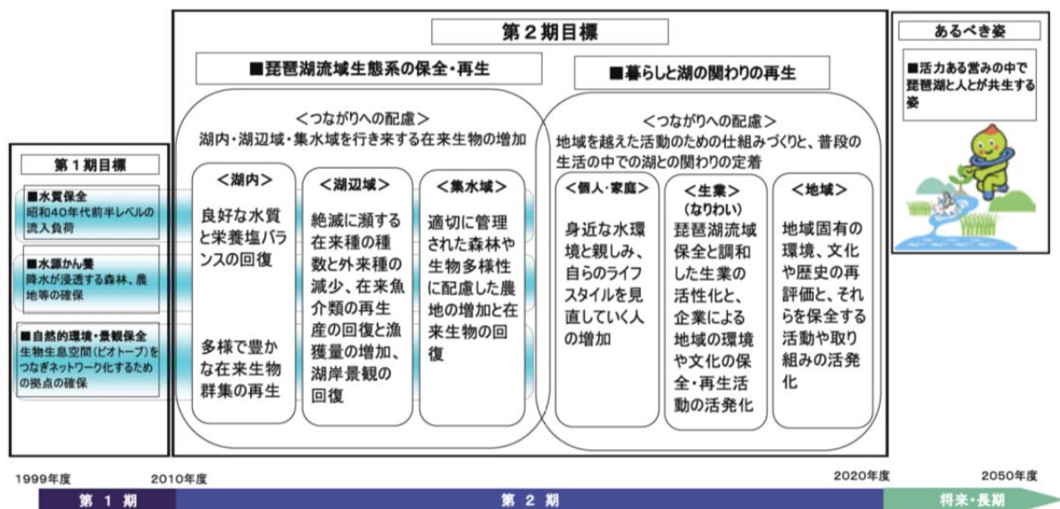
図 3-3-4. 「マザーレイク 21 計画<第 2 期>」段階的計画目標
