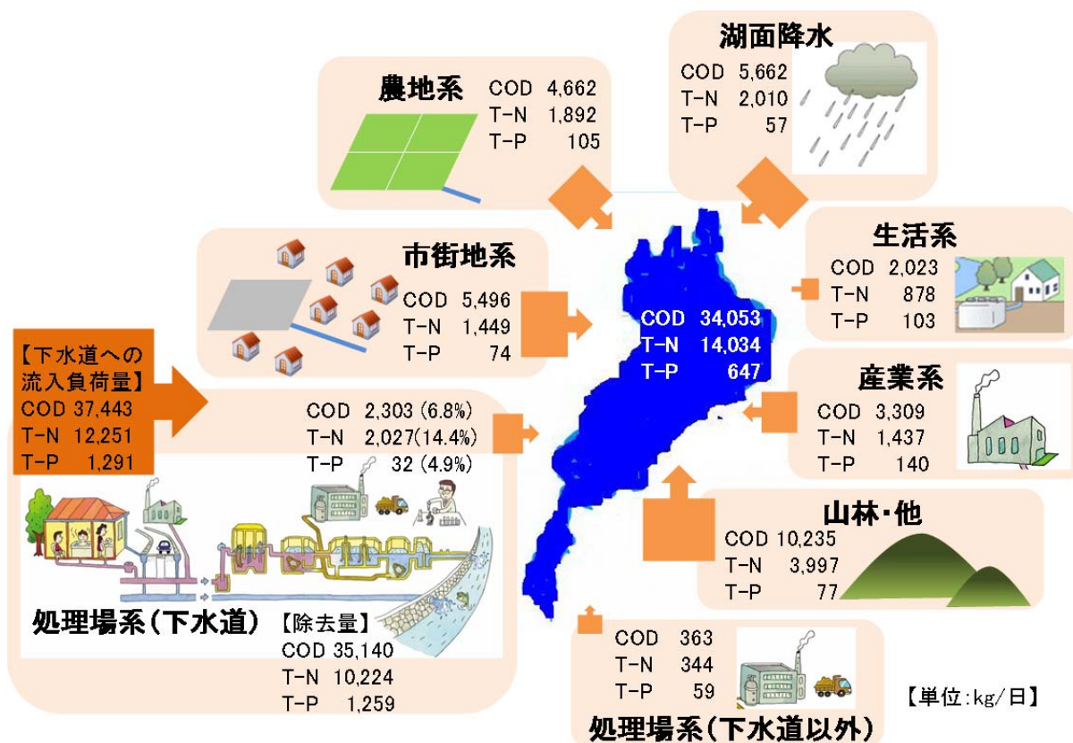
図 3-3-7. 陸域からの流入負荷量 (平成 22 年度)
