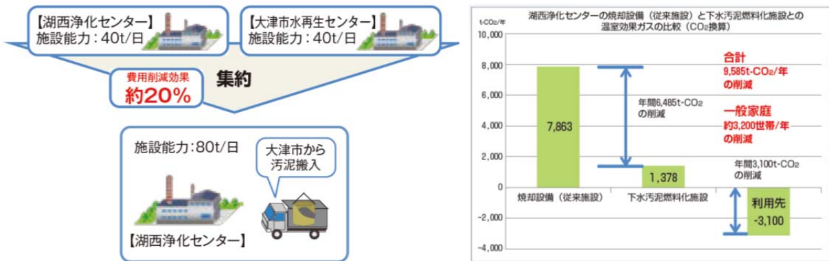
図 3-3-14. 湖西浄化センターにおける污泥処理一括化の効果
