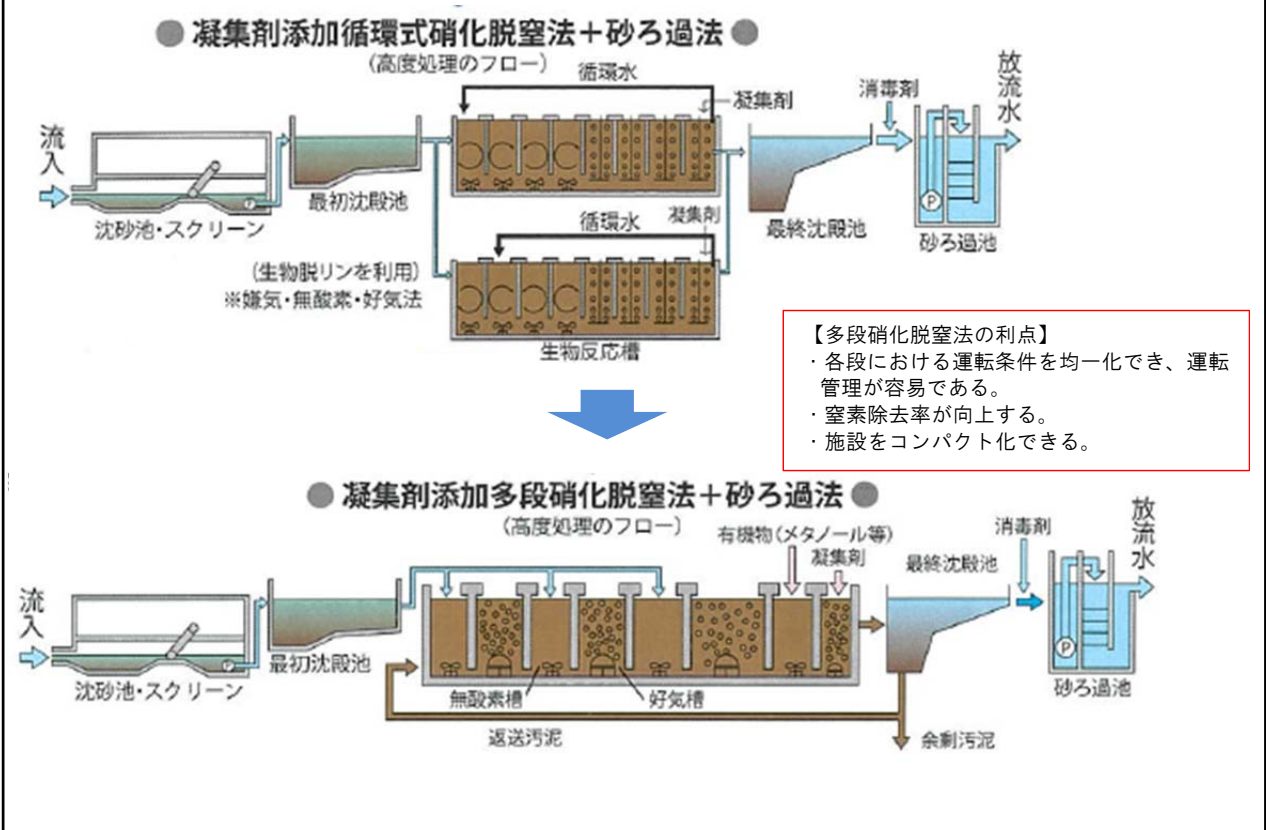
図 3-3-8. 多段硝化脱窒法 (ST 多段法) の概要
