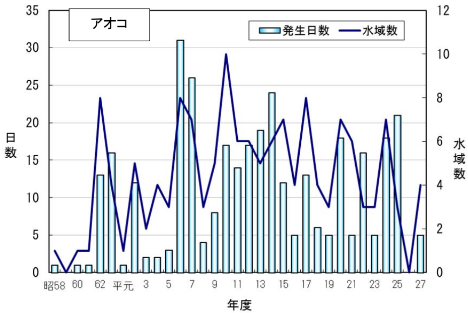
図 3-3-2. 琵琶湖の赤潮・アオコの発生状況の推移
