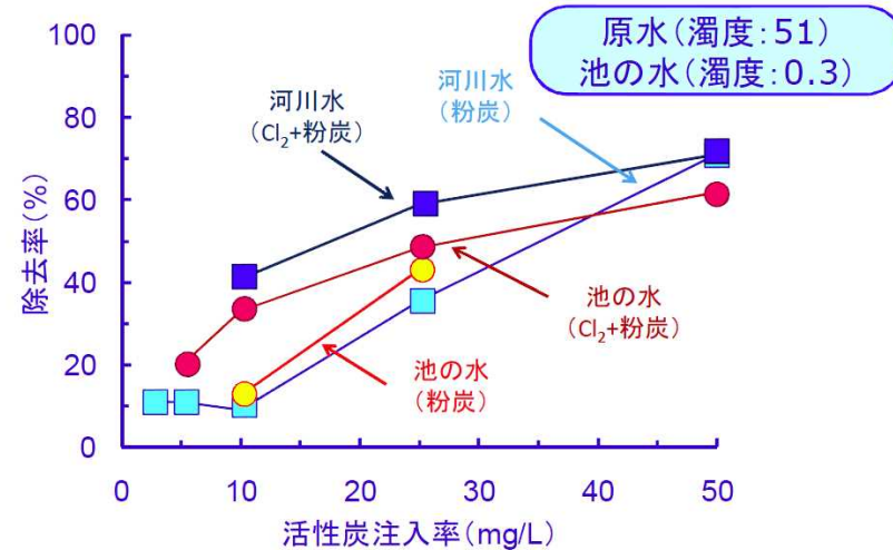
弱塩素処理 + 粉末活性炭で除去率向上 (2011年4~5月, Kosaka et al., Water Research (2012))
