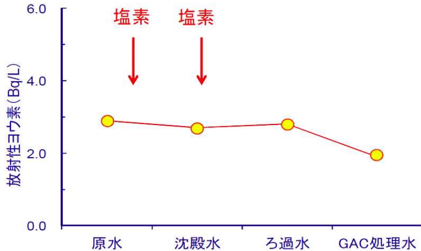
浄水処理工程における放射性ヨウ素の挙動例 (2011年4月, Kosaka et al., Water Research (2012))
