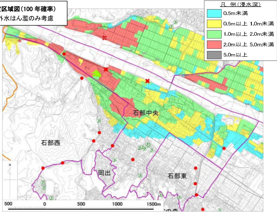
地先の安全度マップ(100年確率) 支川はん濫や内水はん濫も考慮
