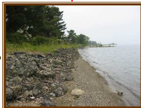
袋詰玉石による浜崖応急処置
