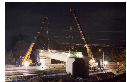
図-10 ランプ橋架設完了
