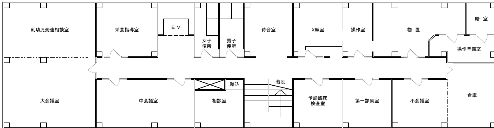
2階平面図
